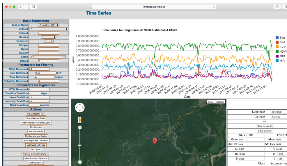
Figura 5. Integração da API WTSS em aplicativos Web.
