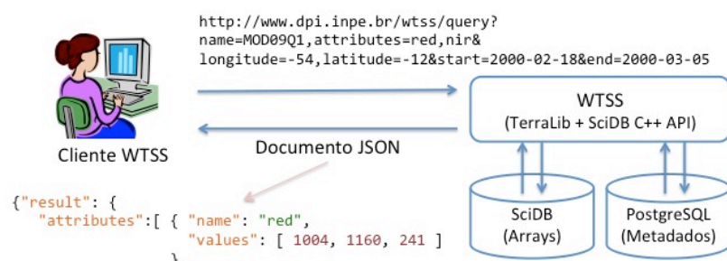
Figura 4. Visão geral da arquitetura do protótipo WTSS.
