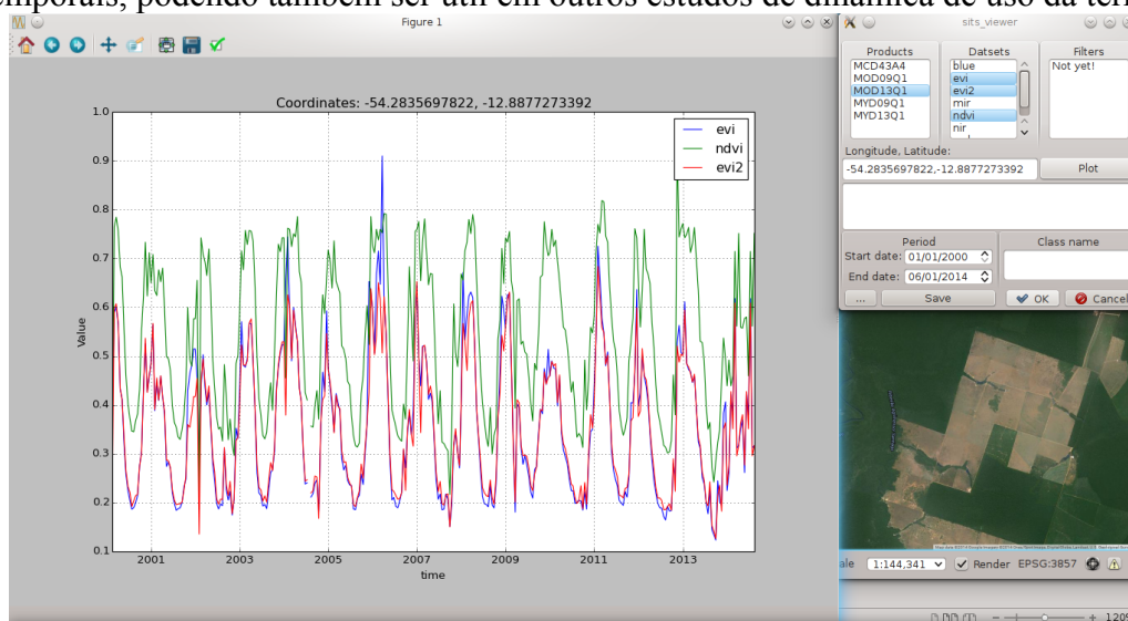
Figura 6. Interface do Plugin SITS Viewer para Quantum GIS.
